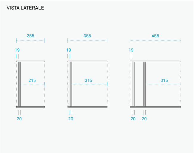
Spazio tecnico e schiena.
