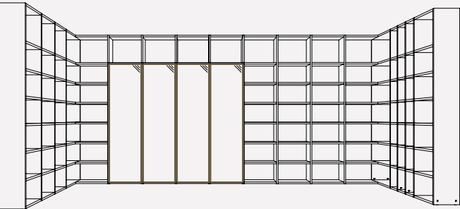
L. 6037 – 2715 – 2416 H. 2626 P. 346
