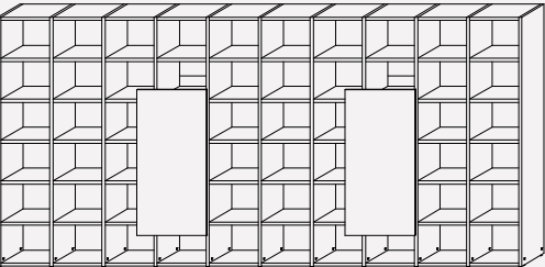
L. 4508 H. 2146 P. 442
