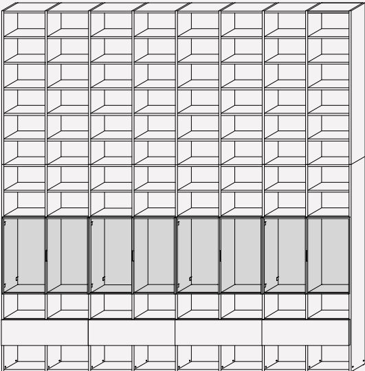
L. 4785 H. 4963 P. 442
