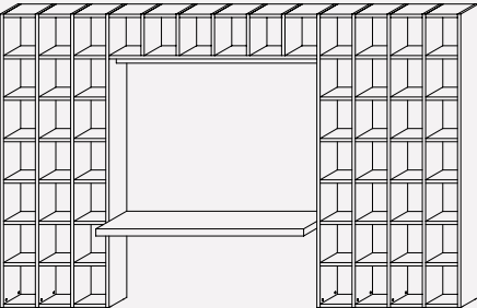
L. 3909 H. 2498 P. 600
