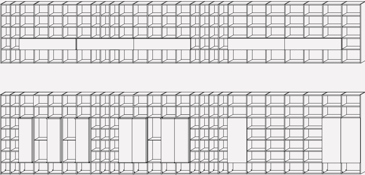
Sopra – Upper composition Sotto – Bottom composition L. 11375 H. 1857 P. 346 L. 11375 H. 2498 P. 346
