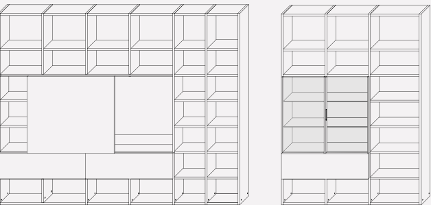
L. 3312 – 1921 H. 2626 P. 346
