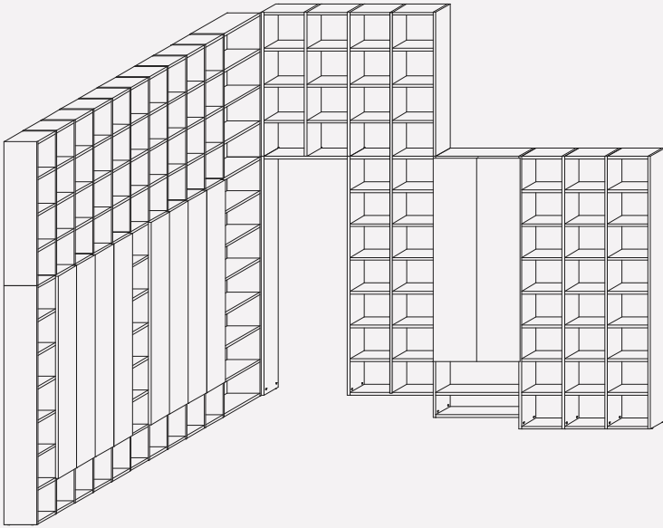
L. 5750 + 4060 H. 3996 – 2846 P. 346
